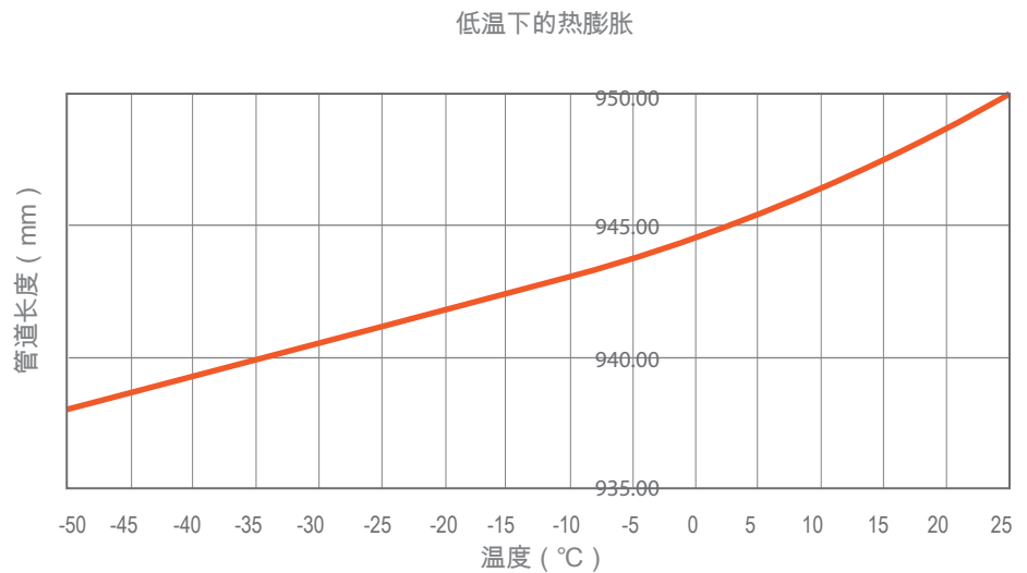
图 2：图表显示了根据泡沫的热膨胀系数预测，温度为 25°C 的 950mm 长的 ZOTEK® F43HT 泡沫在冷却至较低温度时，长度将发生什么变化，
